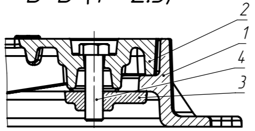
Б-Б (1 : 2.5)
